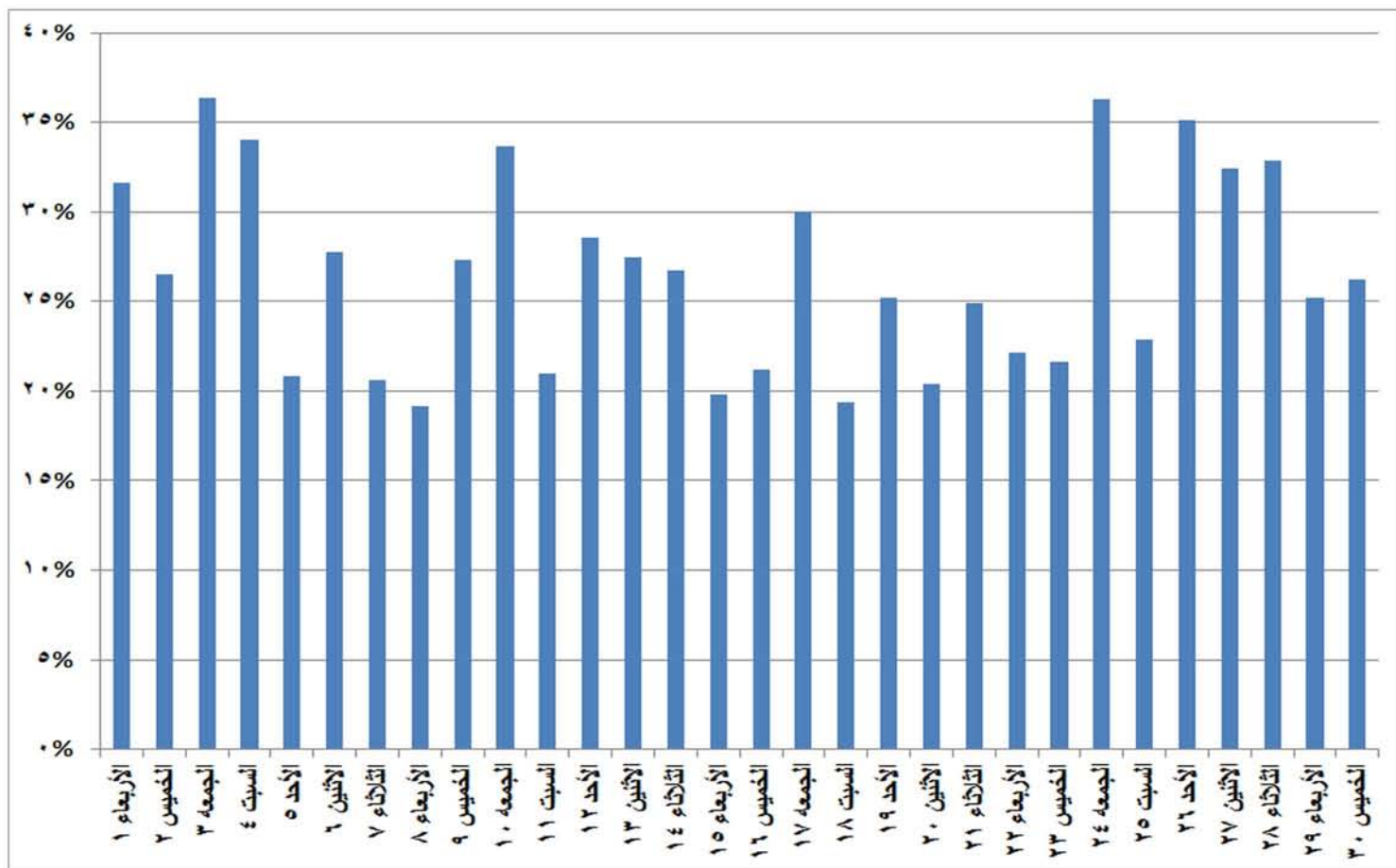
شكل (٢٨) نسب الفائض للحمل الاقصى المسجل يوميا خلال شهر نوفمبر ٢٠١٧
