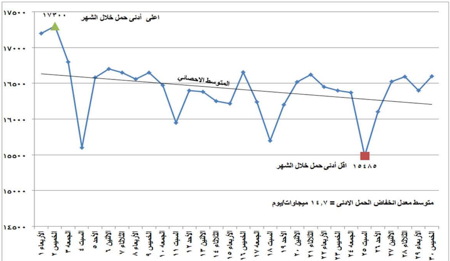
شكل (٢) تطور الحمل الأدنى اليومي خلال شهر نوفمبر ٢٠١٧
