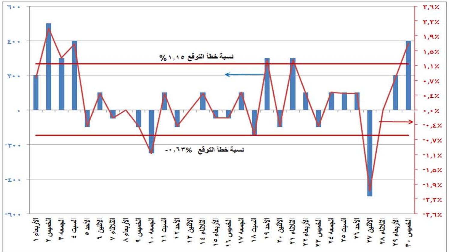
شكل (١٠) الفرق بين الحمل الأقصى المتوقع والمسجل فعلياً ونسبة الفرق إلى الحمل المسجل فعلياً خلال شهر نوفمبر ٢٠١٧
