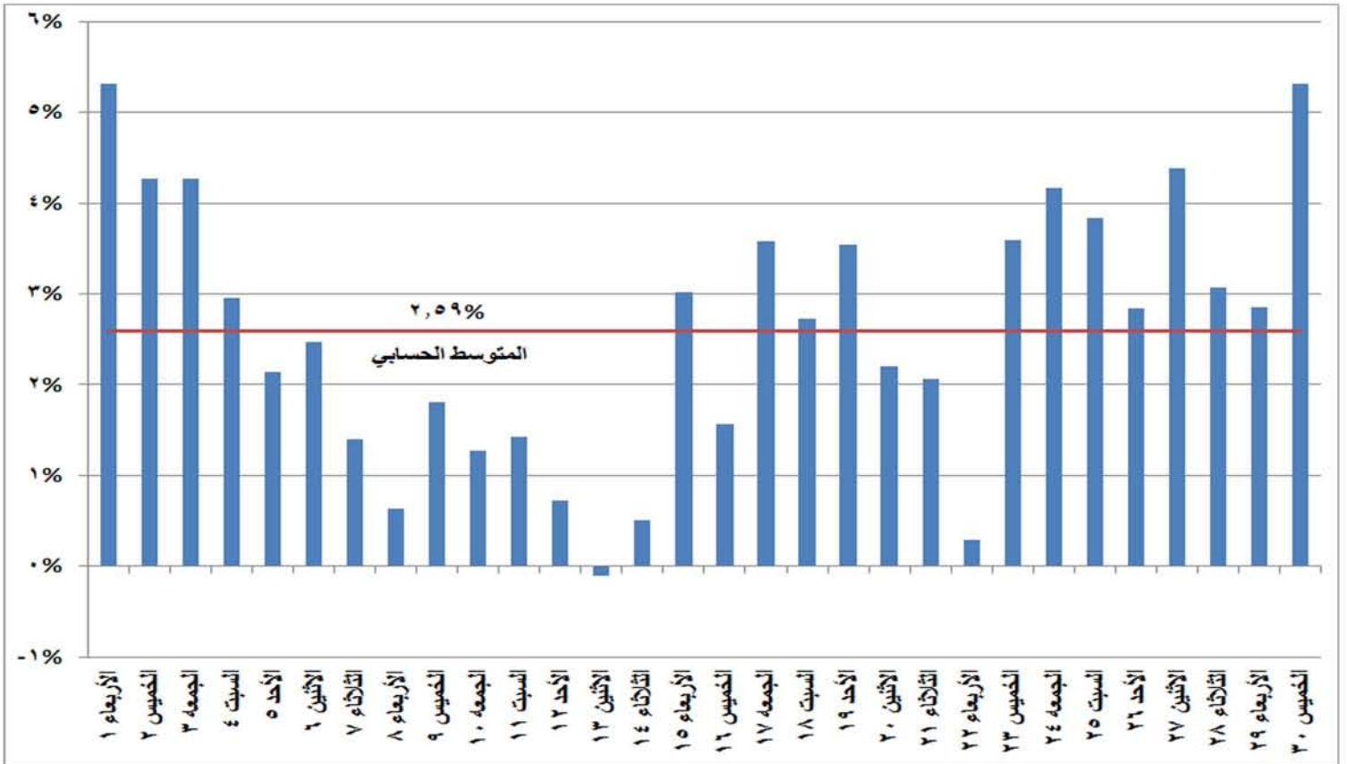
شكل (١٦) نسب التغير في الطاقة الكهربائية المنتجة خلال شهر نوفمبر ٢٠١٧ مقارنة بالشهر المماثل من العام السابق
