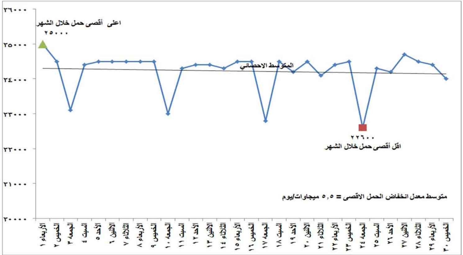
شكل (١) تطور الحمل الاقصى اليومي خلال شهر نوفمبر ٢٠١٧
