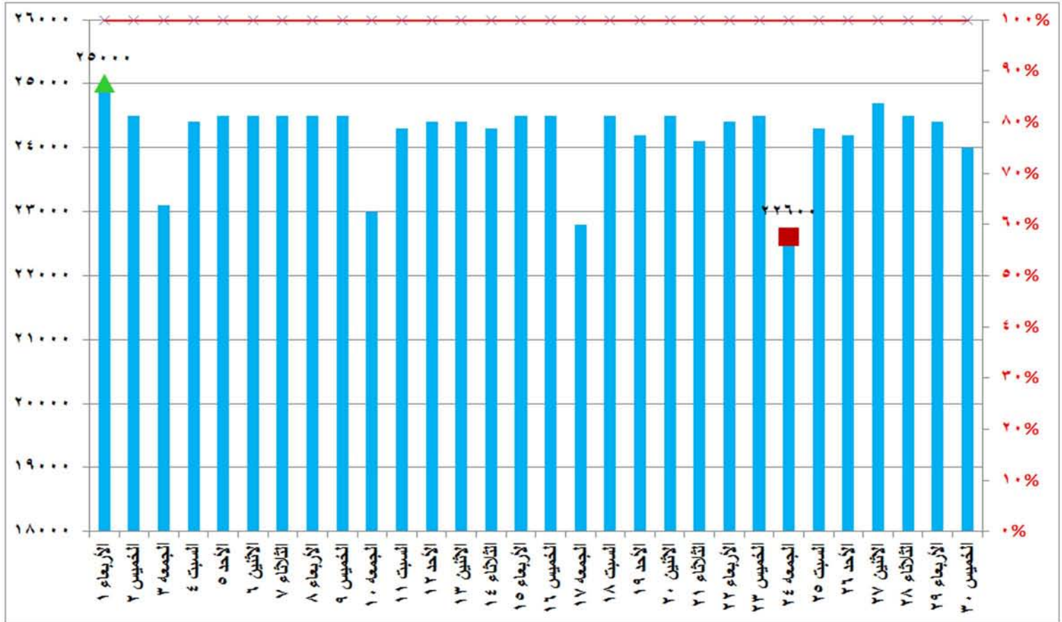
شكل (٥) قدرات الانتاج المتاحة ونسبتها للحمل الأقصى خلال شهر نوفمبر ٢٠١٧
