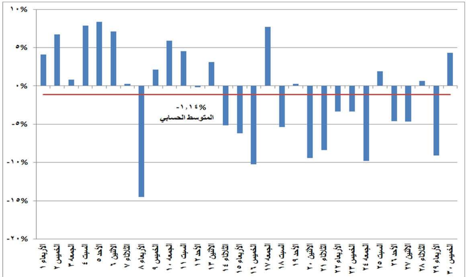
شكل (٢٤) نسب التغير في استخدام المصادر المائية في إنتاج الطاقة الكهربائية خلال شهر نوفمبر ٢٠١٧ مقارنة بالشهر المماثل من العام السابق
