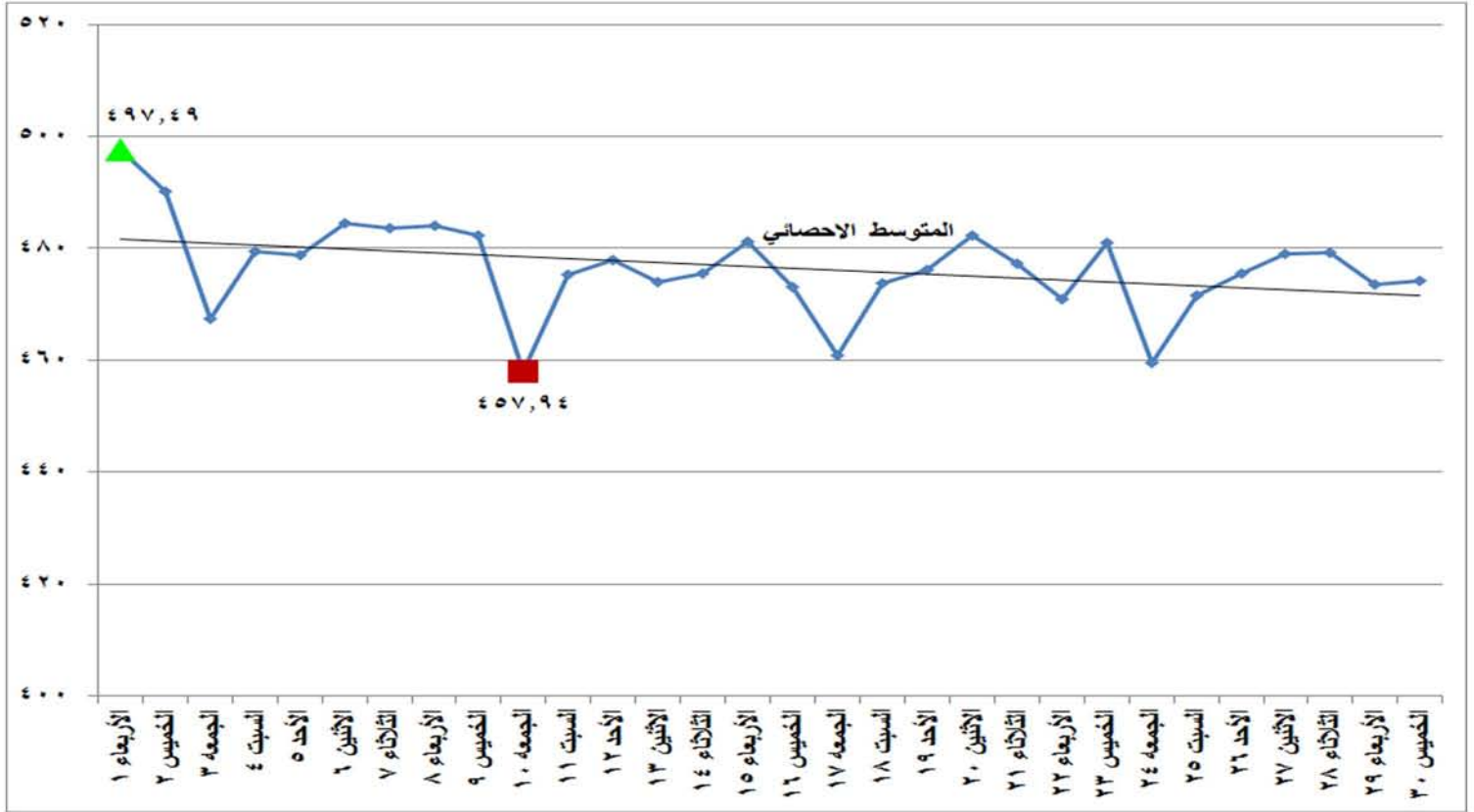
شكل (١٥) إجمالي الطاقة الكهربائية المنتجة من كل المصادر الأولية خلال شهر نوفمبر ٢٠١٧
