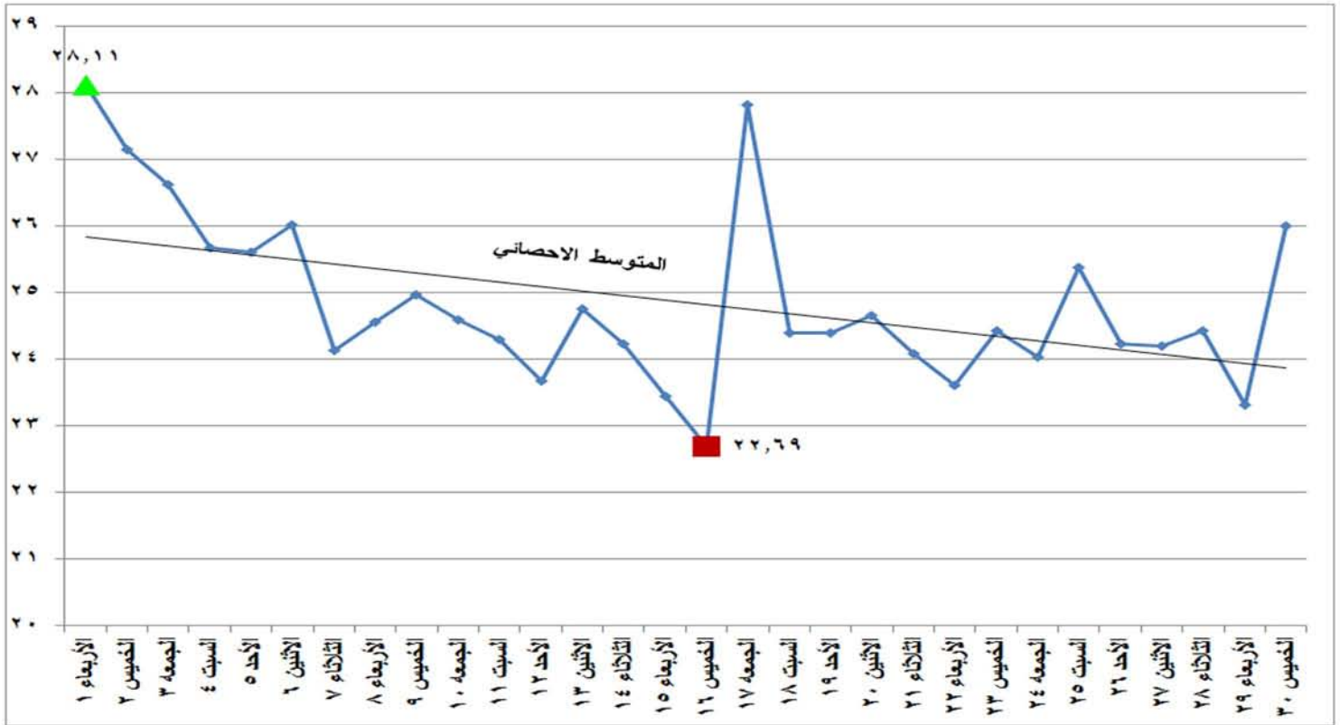
شكل (٢٣) الطاقة الكهربائية المنتجة من المصادر المائية خلال شهر نوفمبر ٢٠١٧
