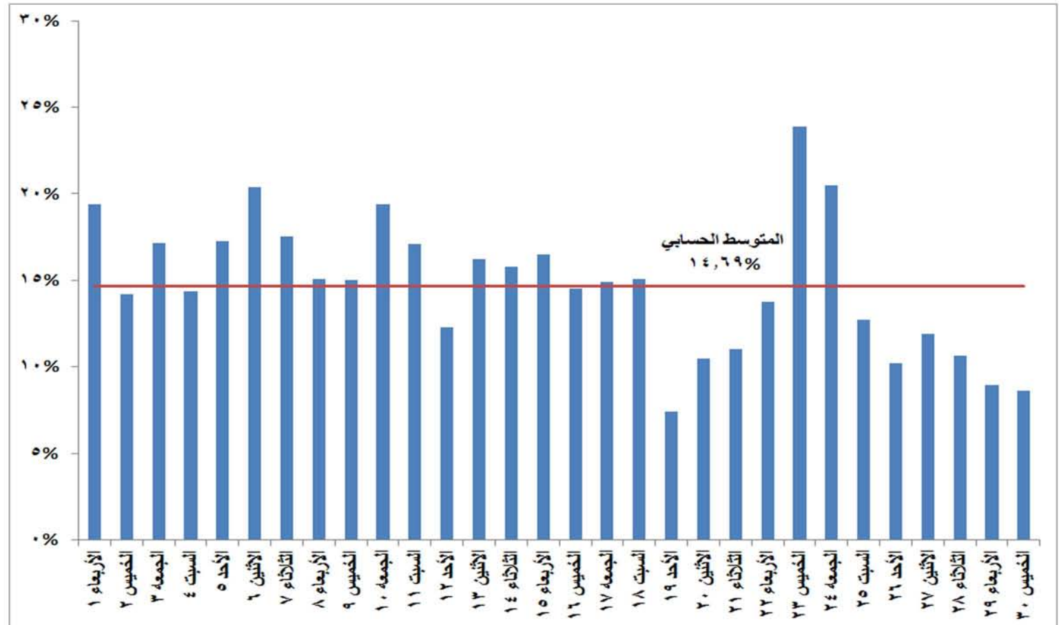
شكل (١٨) نسب التغير في استخدام الغاز الطبيعي في إنتاج الطاقة الكهربائية خلال شهر نوفمبر ٢٠١٧ مقارنة بالشهر المماثل من العام السابق
