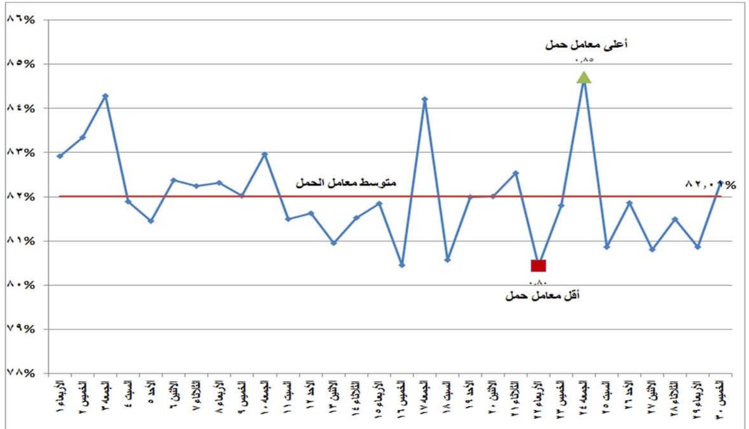
شكل (١٢) إجمالي معامل الحمل لوحدات الانتاج خلال شهر نوفمبر ٢٠١٧
