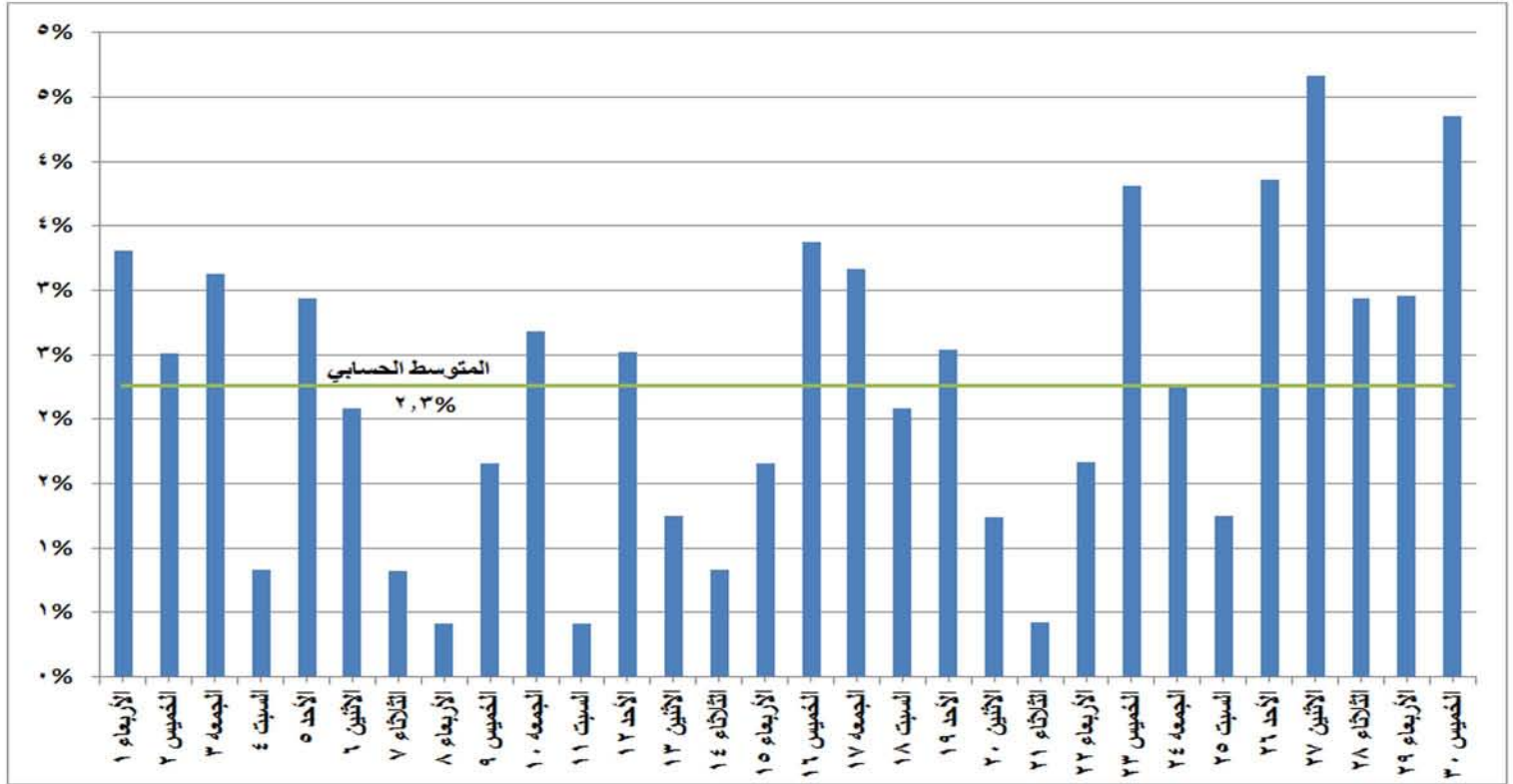
شكل (٩) النسب المئوية للتغير في الحمل الاقصى خلال شهر نوفمبر ٢٠١٧ مقارنة باليوم المماثل من العام الماضي
