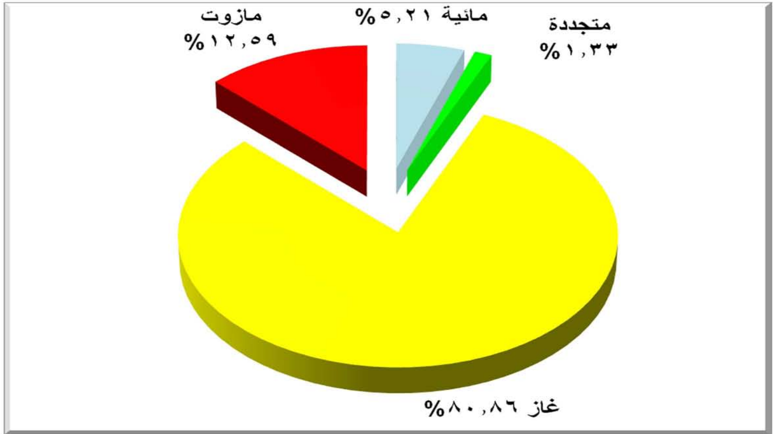
شكل (١٣) متوسط نسب مشاركة مصادر الطاقة الاولية في انتاج الكهرباء خلال شهر نوفمبر ٢٠١٧
