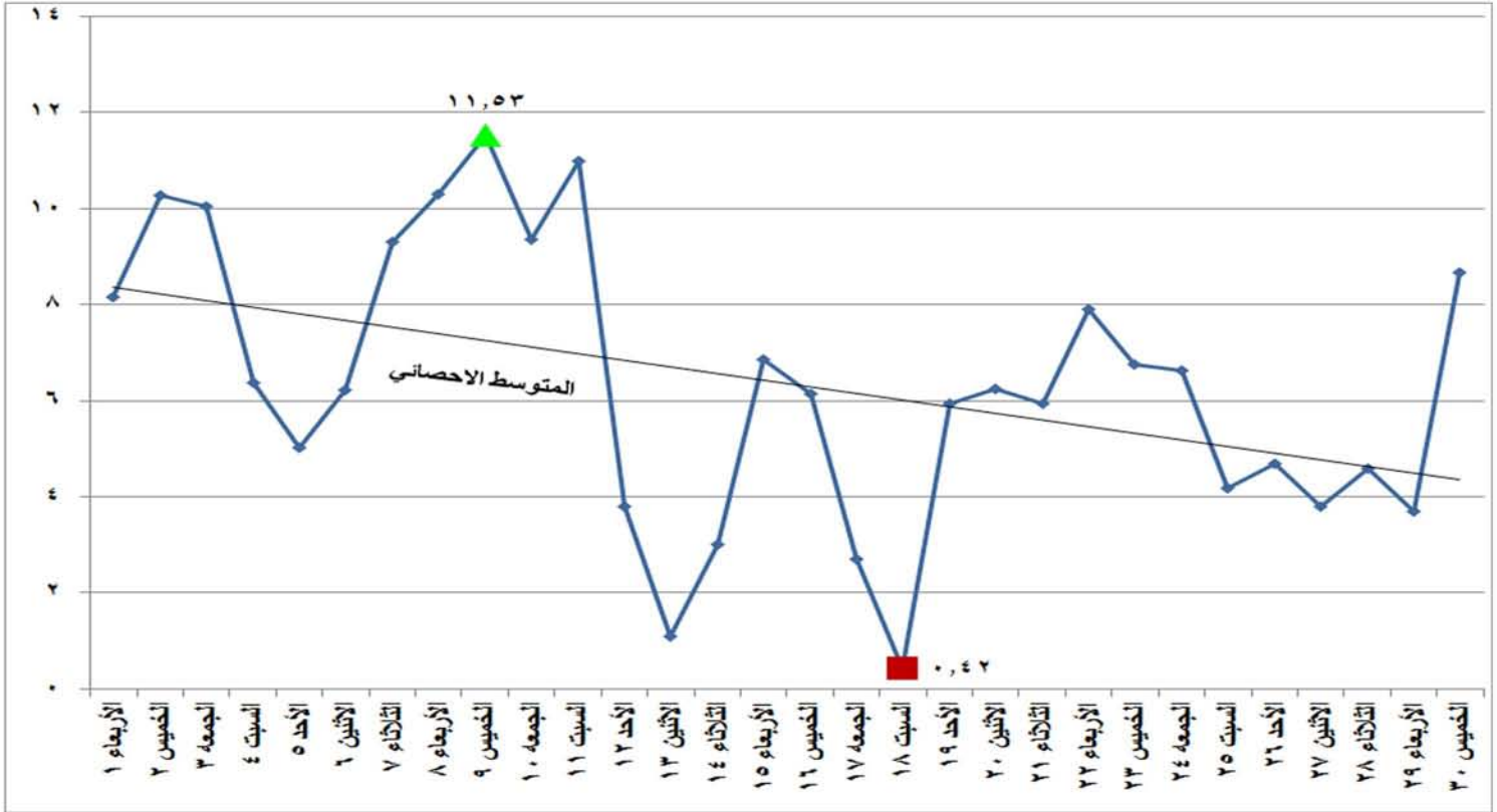
شكل (٢٥) الطاقة الكهربائية المنتجة من الرياح والشمس خلال شهر نوفمبر ٢٠١٧
