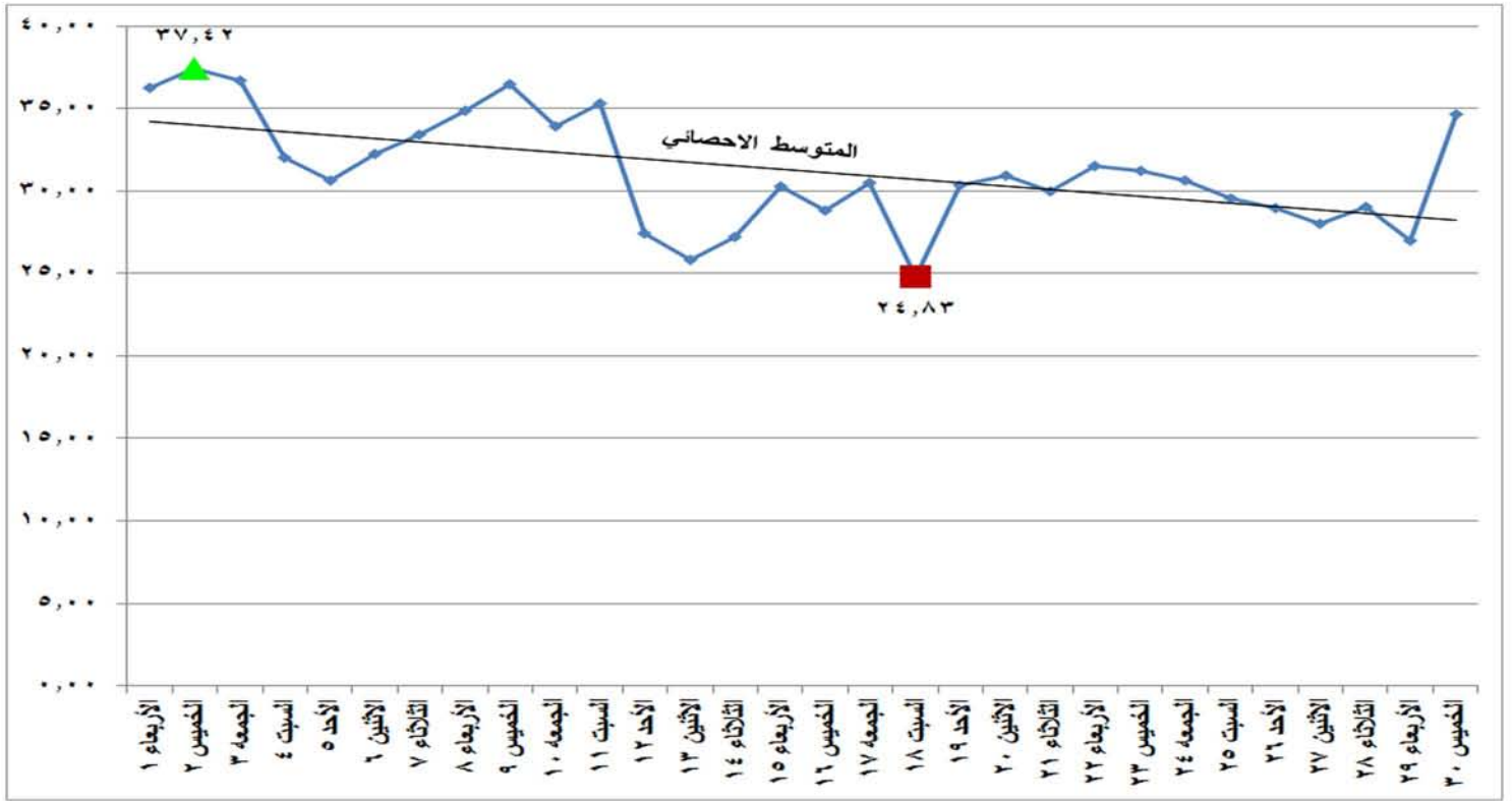
شكل (٢١) الطاقة الكهربائية المنتجة من المصادر غير الحرارية خلال شهر نوفمبر ٢٠١٧
