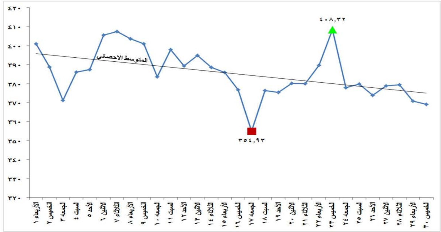
شكل (١٧) الطاقة الكهربائية المنتجة من الغاز الطبيعي خلال شهر نوفمبر ٢٠١٧
