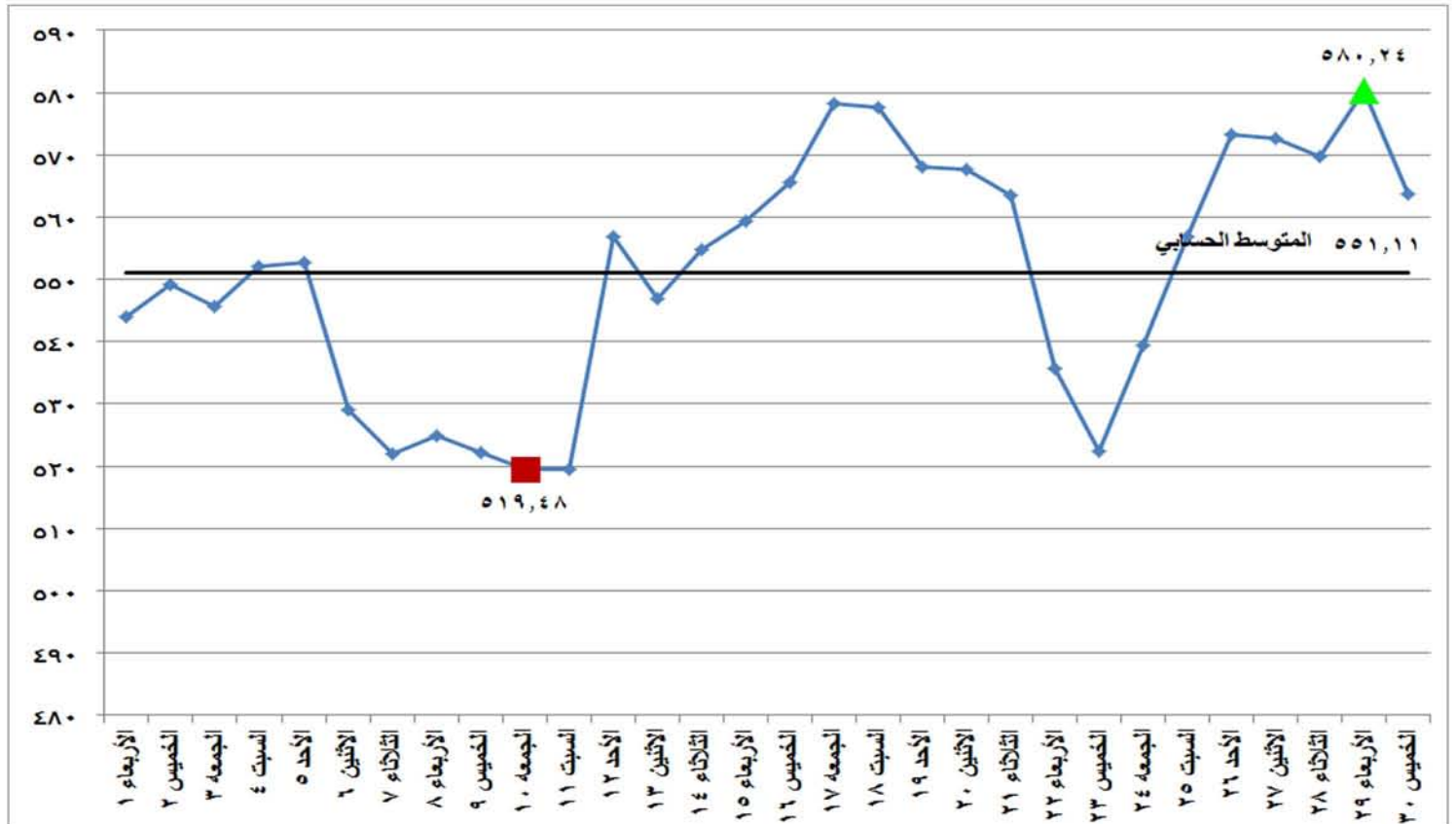
شكل (١٤) معامل انبعاثات غاز ثاني اكسيد الكربون المكافئ على مدى شهر نوفمبر ٢٠١٧
