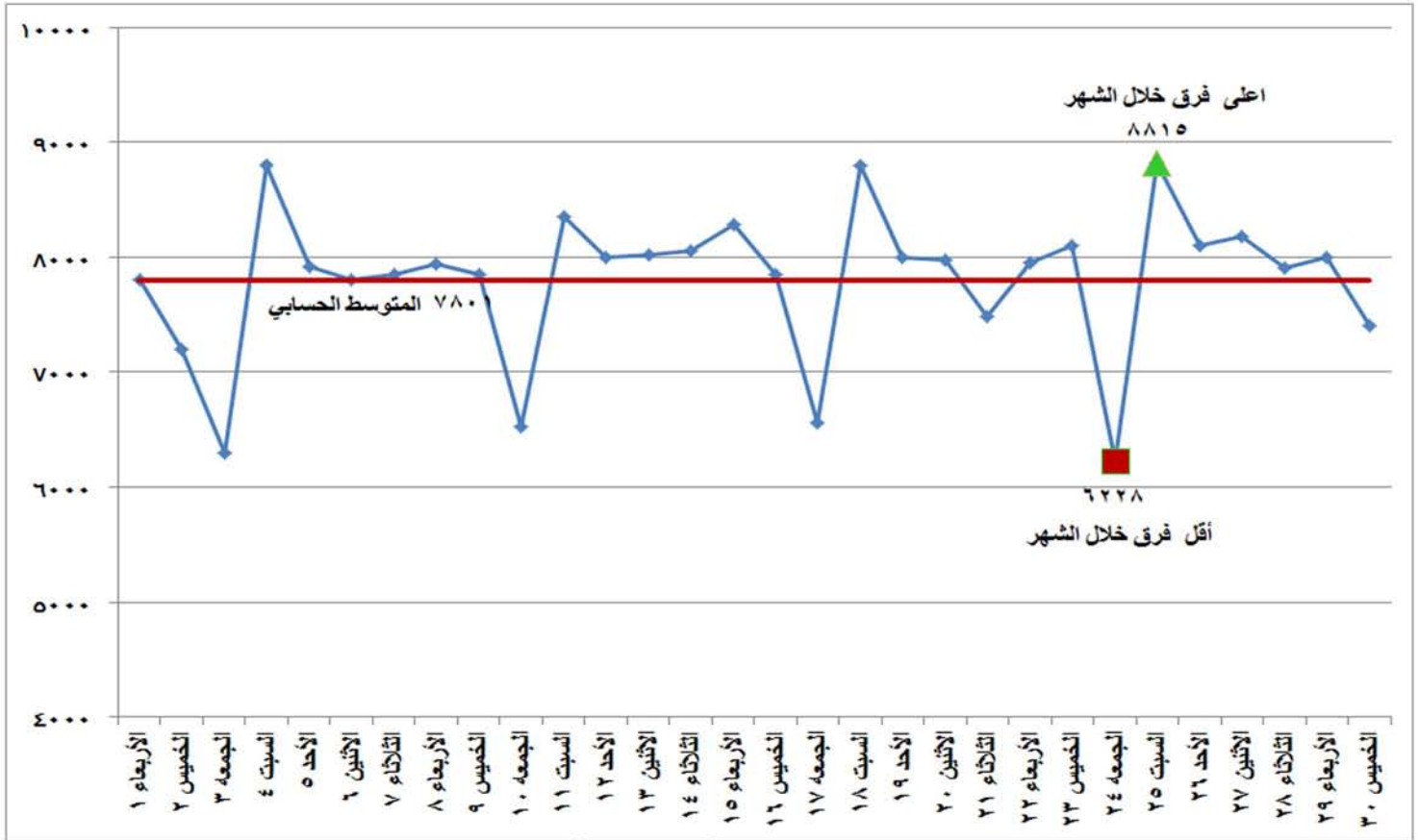
شكل (٣) الفرق بين أقصى وأدنى حمل خلال شهر نوفمبر ٢٠١٧
