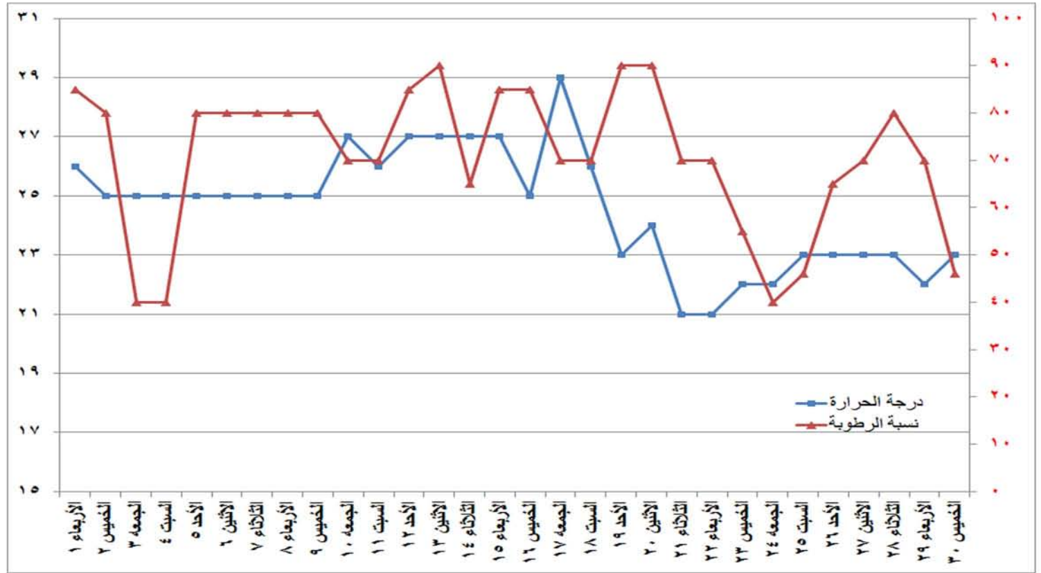
شكل (١١) التغيير في درجة الحرارة والرطوبة النسبية خلال شهر نوفمبر ٢٠١٧
