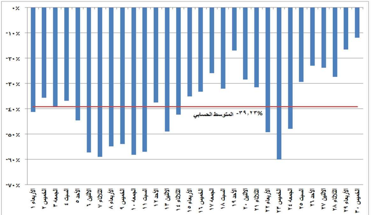
شكل (٢٠) نسب التغير في استخدام المازوت في إنتاج الطاقة الكهربائية خلال شهر نوفمبر ٢٠١٧ مقارنة بالشهر المماثل من العام السابق
